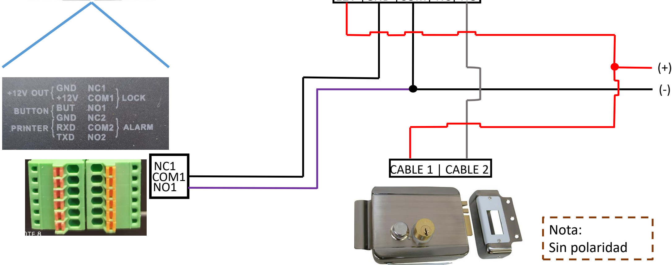
Cerradura Electromecánica
